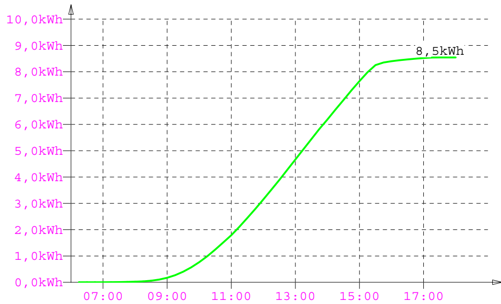
eingespeiste Energie
