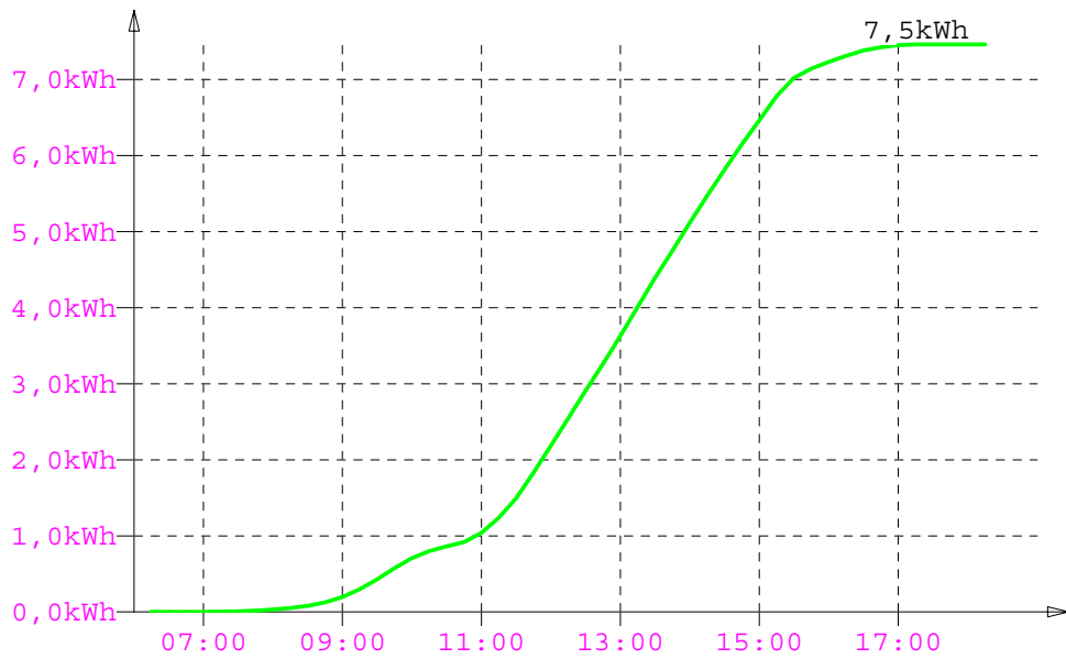
eingespeiste Energie
