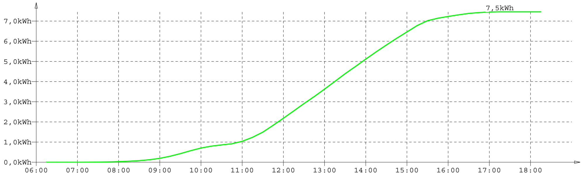
eingespeiste Energie
