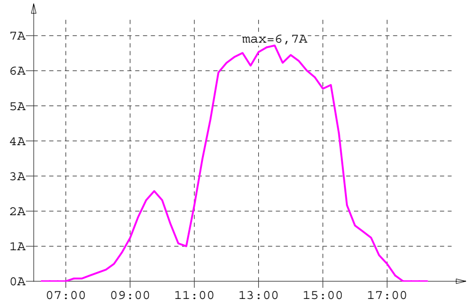
Netzstrom
