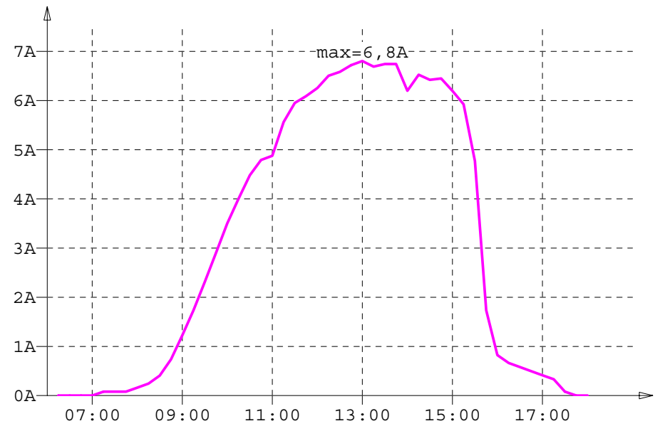
Netzstrom
