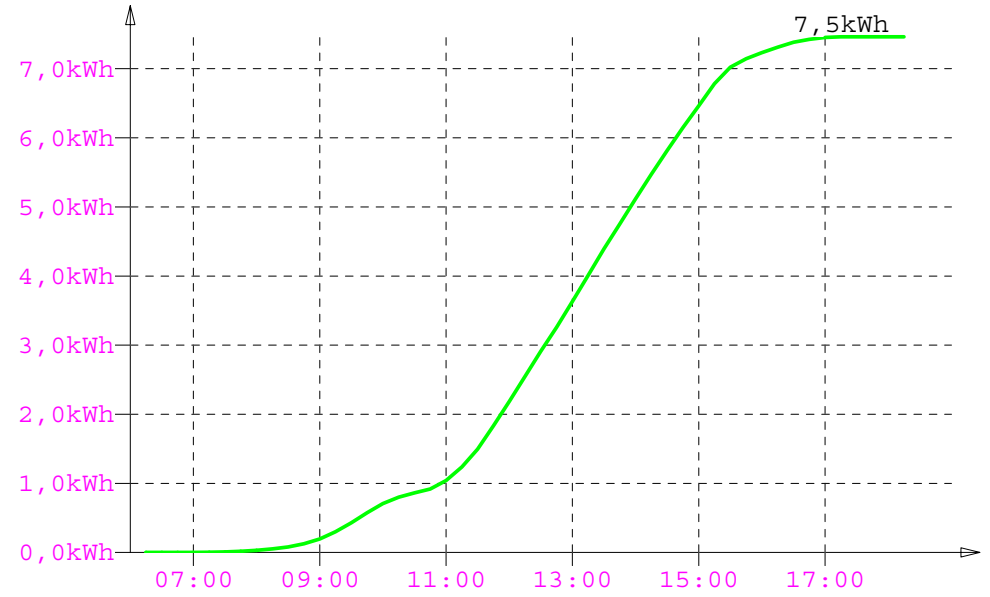
Netzstrom
