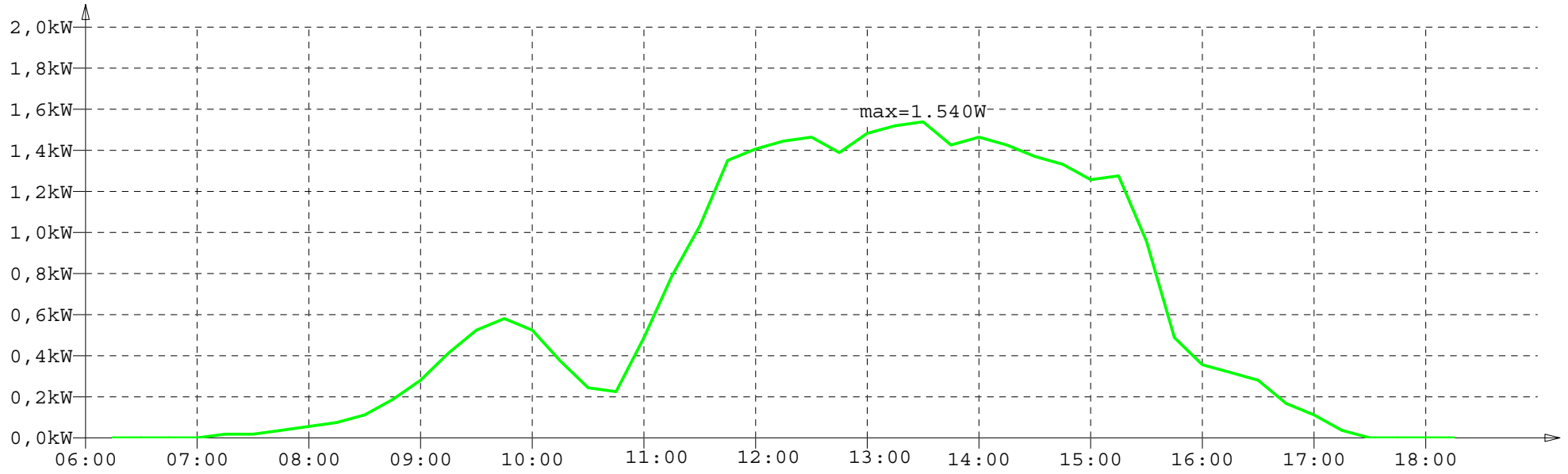
eingespeiste Energie
